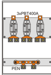
ZK-2a 400A
