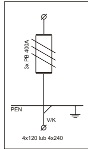
ZK-2a 400A
