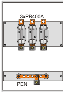
ZK-1a 400A
